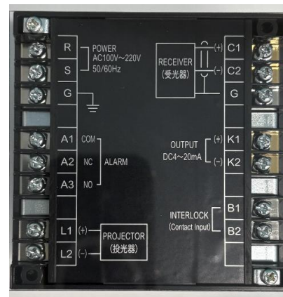
②配線部
